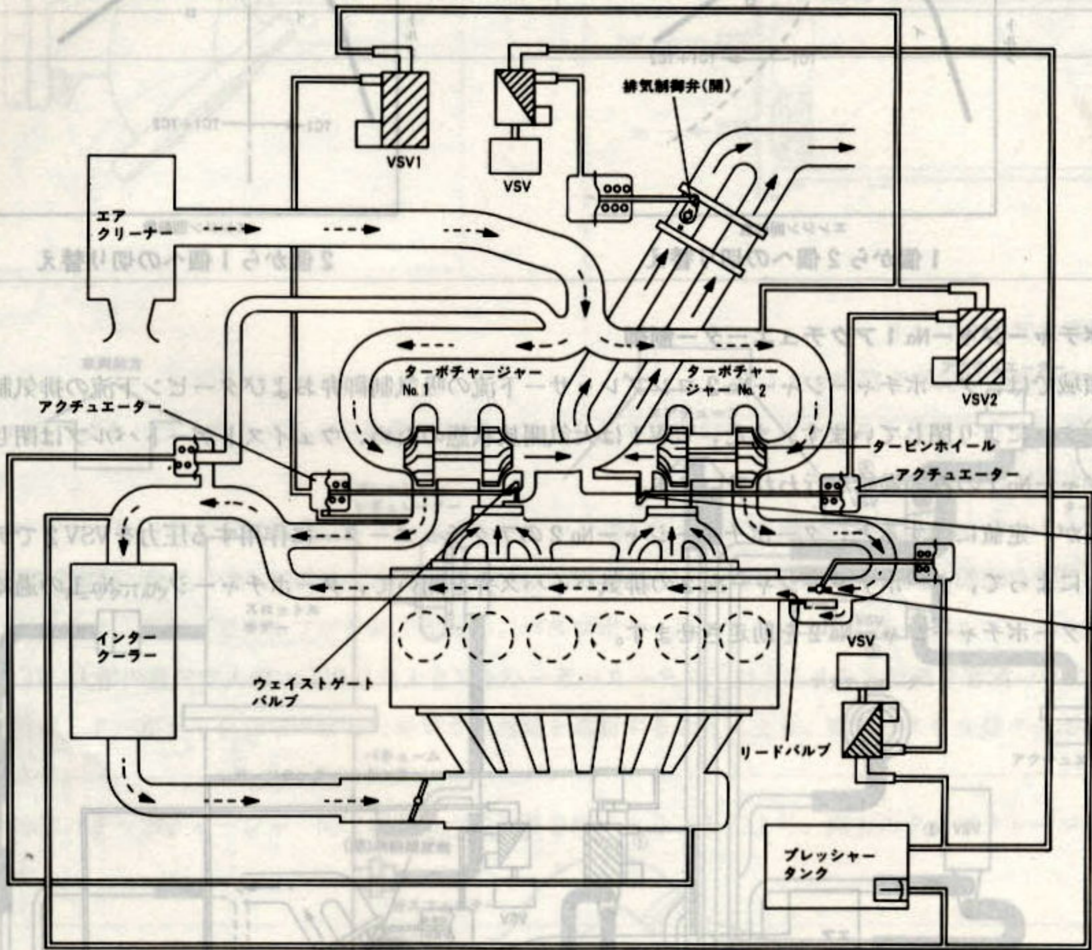
ターボチャージャーNo. 1 + No. 2 による過給
